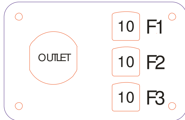
kytkinpaneeli, sekä sulakkeet ja 12V-ulosotto hanskalokerossa.
