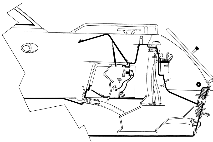
Kuva 4. Tyhjennysjärjestelmä
